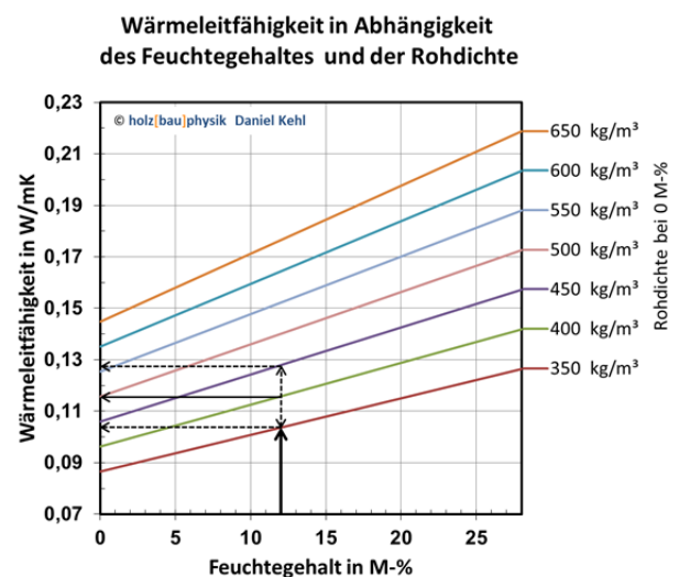
Abb. 1: Abhängigkeit der Wärmeleitfähigkeit des Holzes (quer zur Faser) von der Rohdichte und dem Feuchtegehalt
